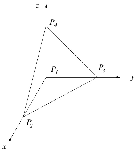
FIG. 4.13 – un tétraèdre
