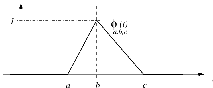
FIG. 3.2 – Fonction « chapeau »
